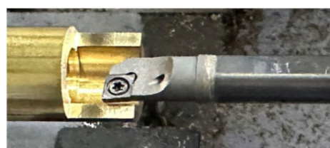
小物部品加工用ボーリングバー 最小加工径 9mm
